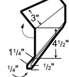
LG 130 SLIDING DOOR DRIP CAP
